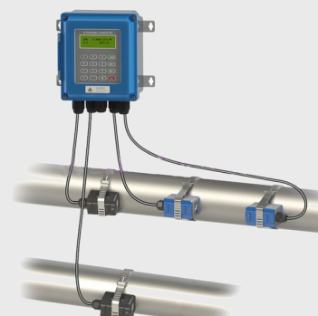
Compteur d'énergie non intrusif
